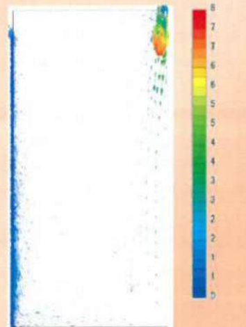
気流分布シミュレーション結果
